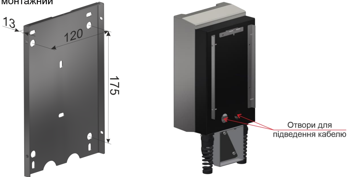
Рис.5 - Монтажний кронштейн для кріплення ЗС Рис.6 - Можливість підведення кабелю живлення з тильної сторони зарядної станції
