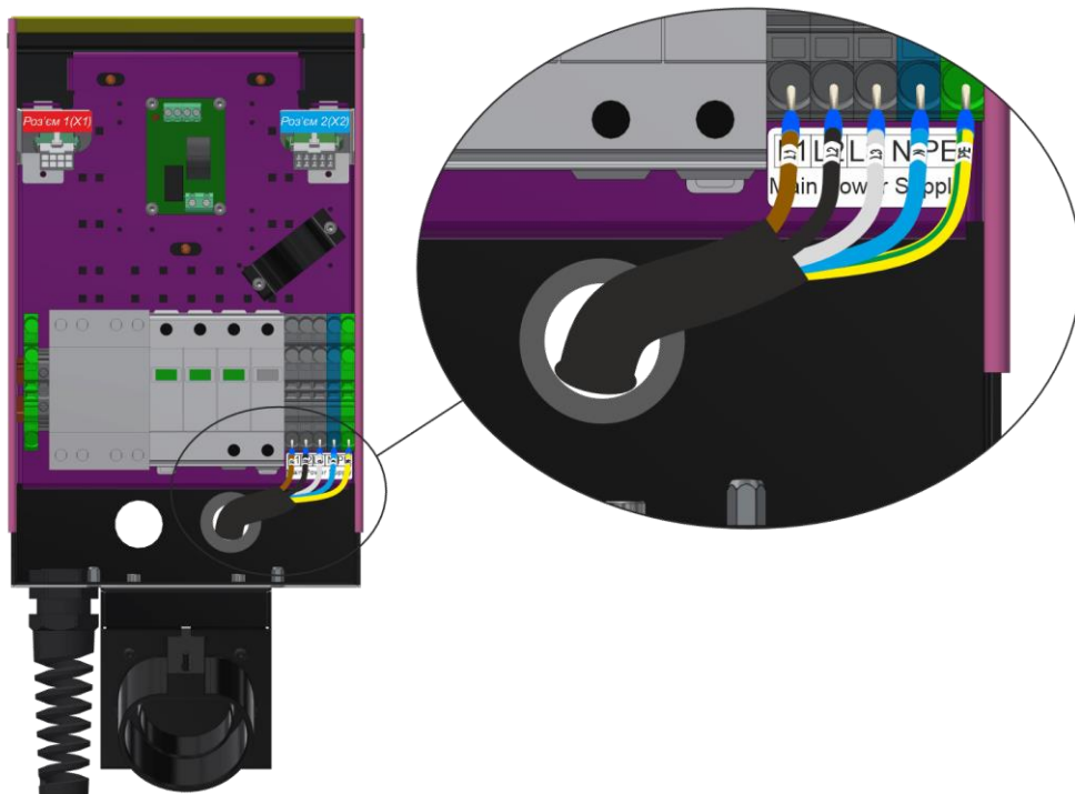
Рис.12 – Підключення кабелю живлення
