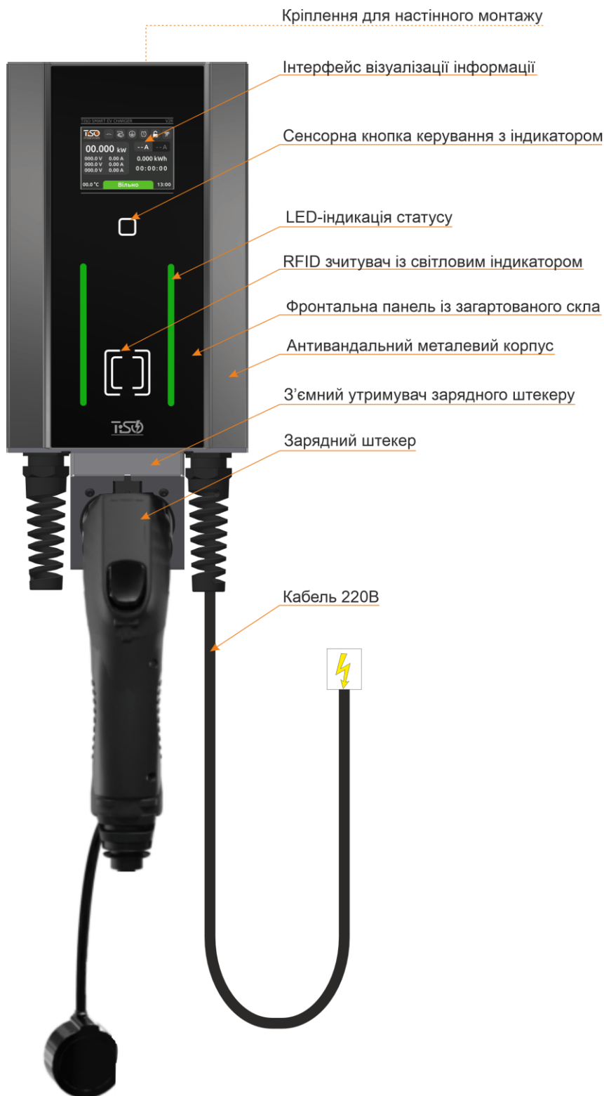
Рис.2 – Загальний вигляд станції
