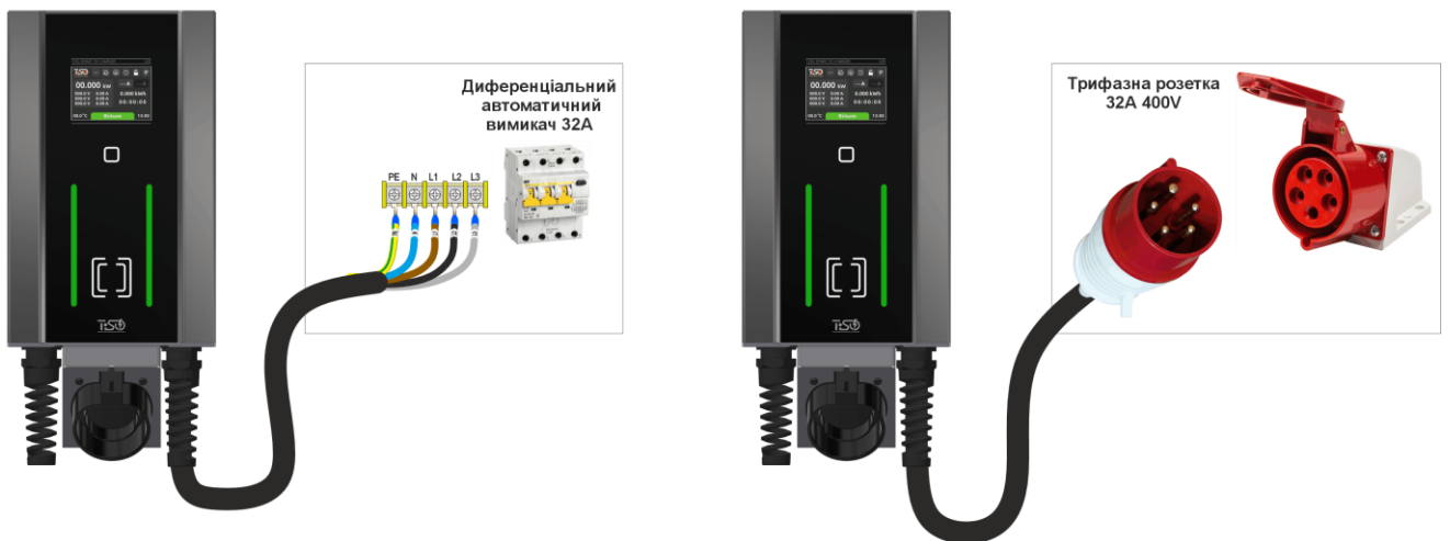
Рис. 9 – Варіанти підключення трьохфазної ЗС
