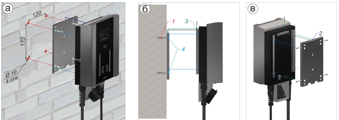
Рис.7 – Монтаж зарядної станції на стіну
