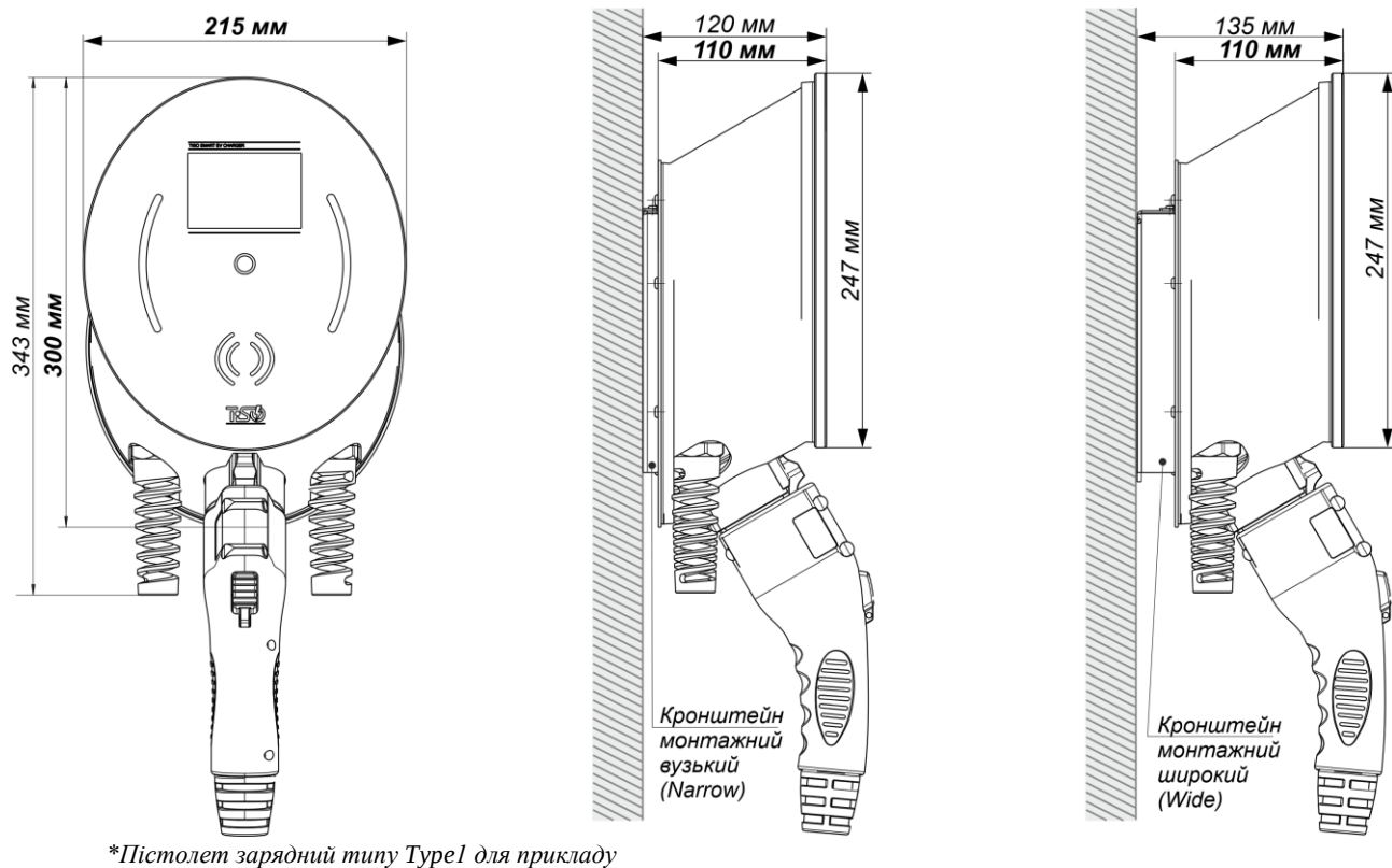
Рис.12 - Габарити та загальний розмір зарядного пристрою для електроавтомобіля
