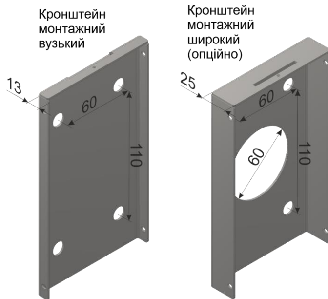
Рис. Рекомендації щодо габаритів монтажу на стіну
